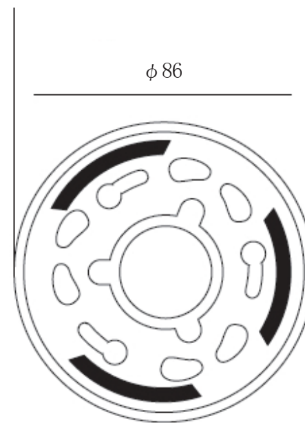
(設置面)
